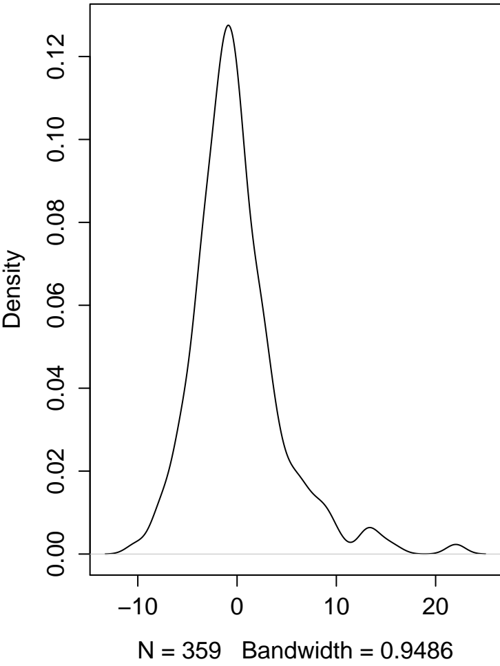
density.default(x = res)
