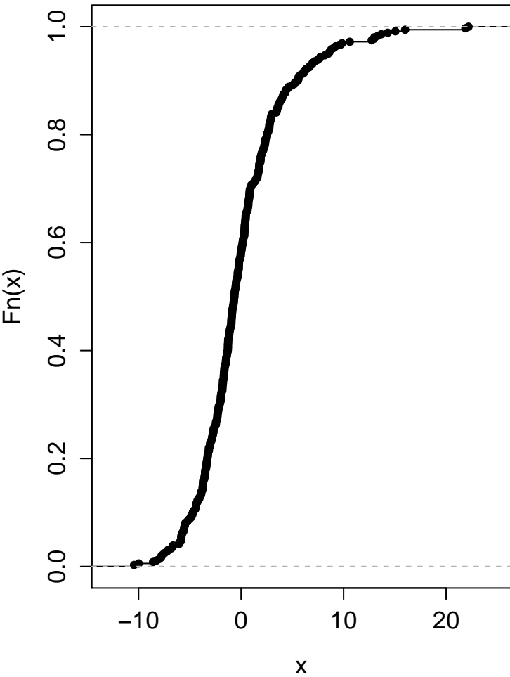
ecdf(res)
