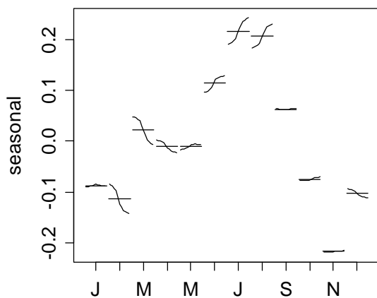
Monthplot, s.window=13
