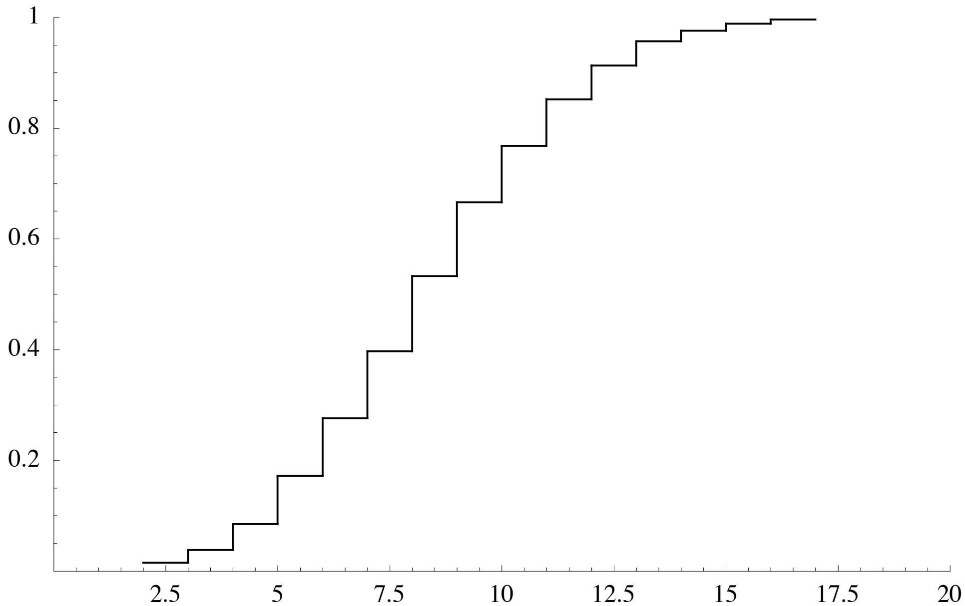
Radioaktiver Zerfall von Am – 241 : empirische Verteilungsfunktion
