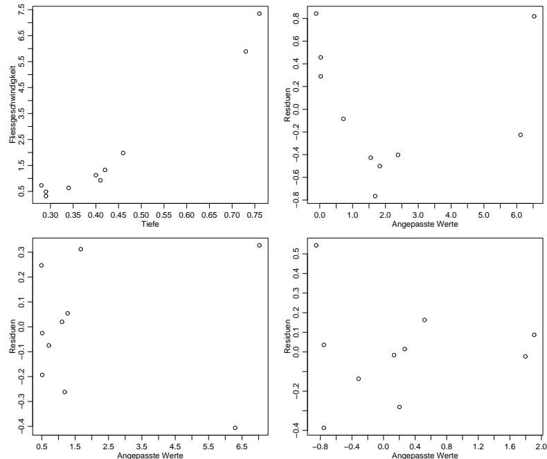
Abbildung 5.4: Streudiagramm von Tiefe und Fließgeschwindigkeit (oben links), Tukey-Anscombe Plots für einfache lineare Regression (oben rechts), für quadratische Regression (siehe Kapitel 5.3.1) (unten links) und für einfache lineare Regression mit logarithmierten Variablen \log(Y) und \log(x) (unten rechts).
