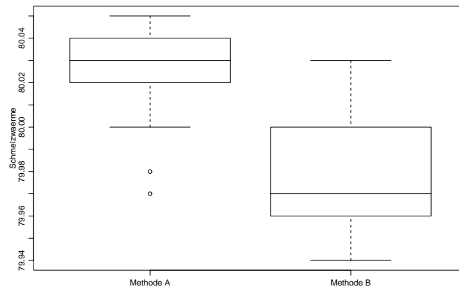
Abbildung 4.1: Boxplots für die zwei Methoden zur Bestimmung der Schmelzwärme von Eis.
