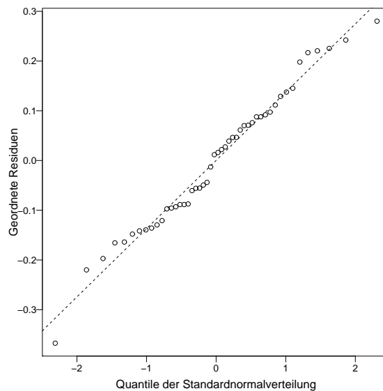
Abbildung 4.3.c: Normal plot der Residuen für das Beispiel der Sprengungen.
