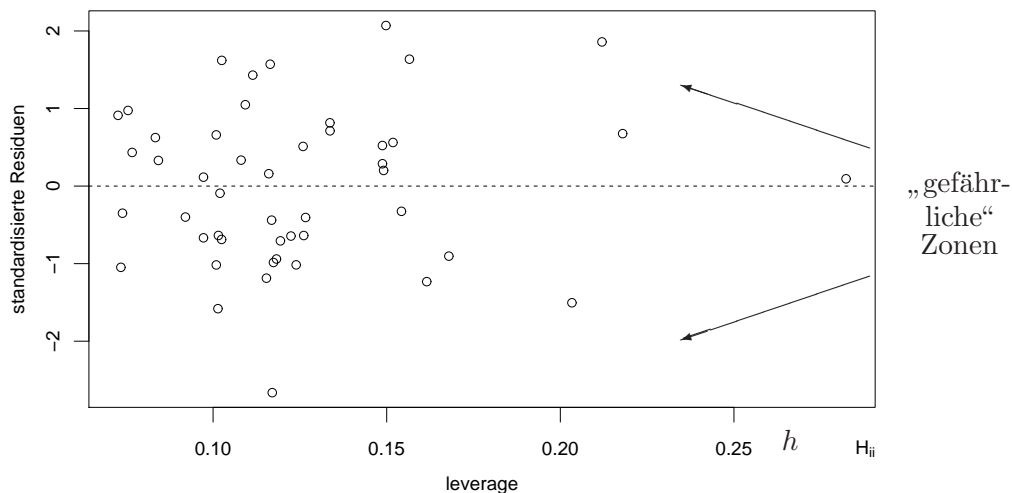
Abbildung 4.10.c: Hebelarm-Diagramm für das Beispiel der Sprengungen
